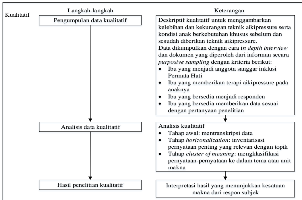
Gambar 2. Tahapan penelitian
